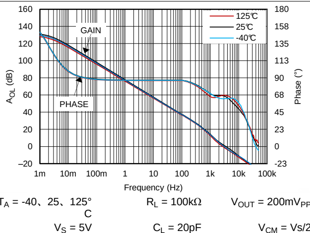
Figure 29. 开环增益和相位, 5V, 100kΩ 负载
