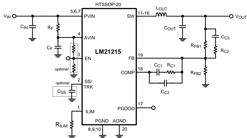
简化应用电路
