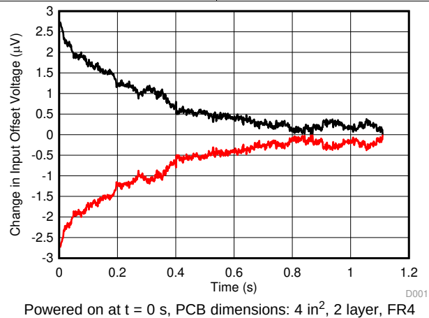
图 53. Warm-Up Time
