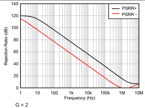
图 26. PSRR vs Frequency (RTI)
