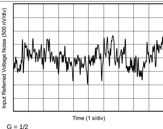
图 35. 0.1-Hz to 10-Hz RTI Voltage Noise
