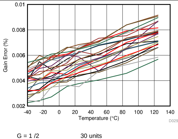
图 29. Gain Error vs Temperature
