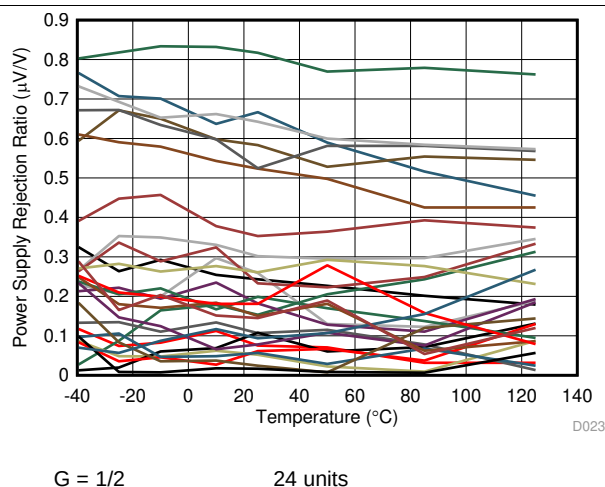
图 23. PSRR vs Temperature
