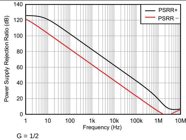
图 25. PSRR vs Frequency (RTI)
