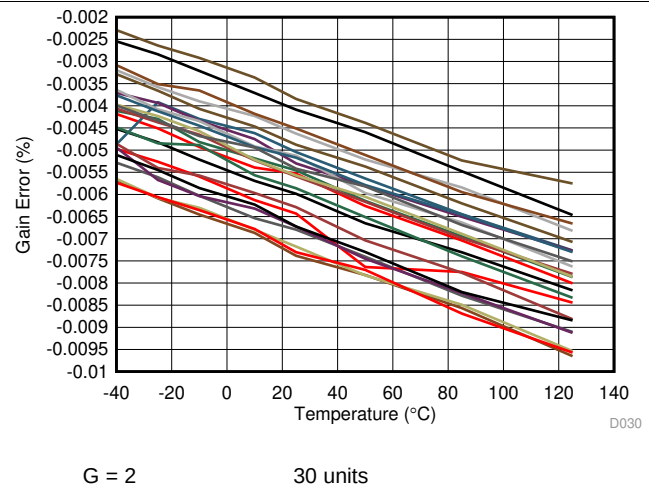
图 30. Gain Error vs Temperature
