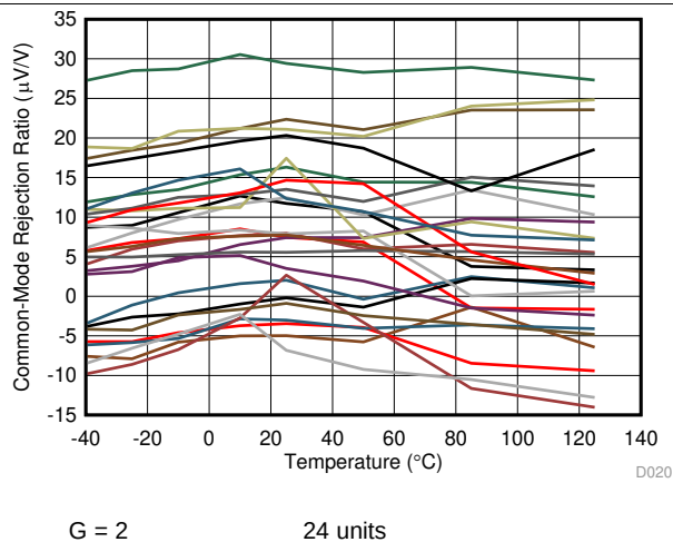
图 20. CMRR vs Temperature
