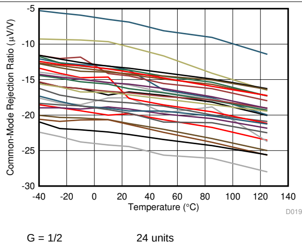
图 19. CMRR vs Temperature
