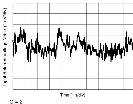
图 36. 0.1-Hz to 10-Hz RTI Voltage Noise
