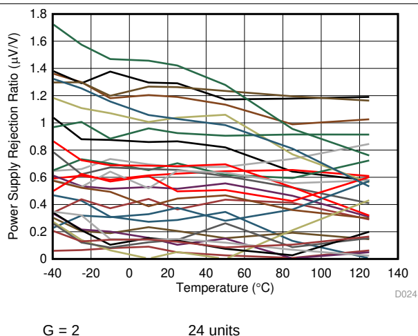
图 24. PSRR vs Temperature
