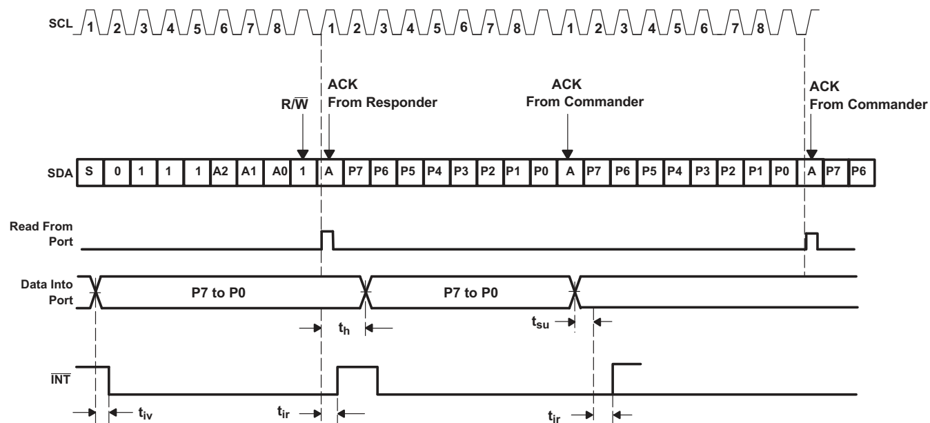
图 8-2. Read Mode (Input)
