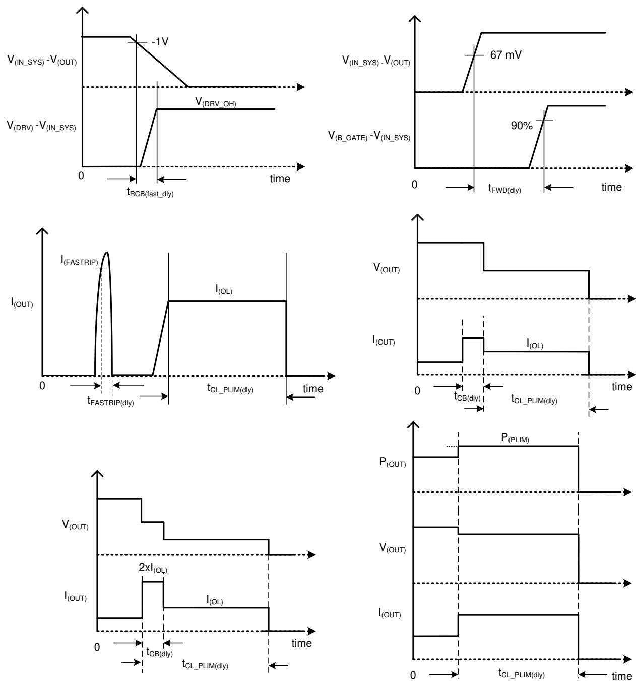
图 20. Timing Waveforms
