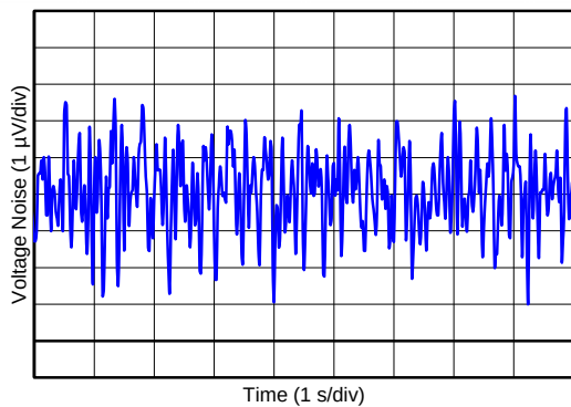
图 11. 0.1-Hz to 10-Hz Input Voltage Noise
