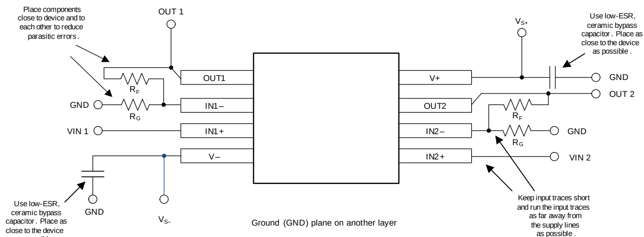
图 41. Layout Example
