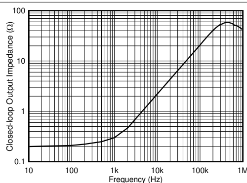
图 7-6. Output Impedance vs. Frequency
