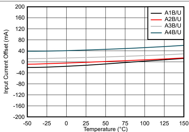
图 7-2. TMCS1107-Q1 Input Offset Current vs. Temperature
