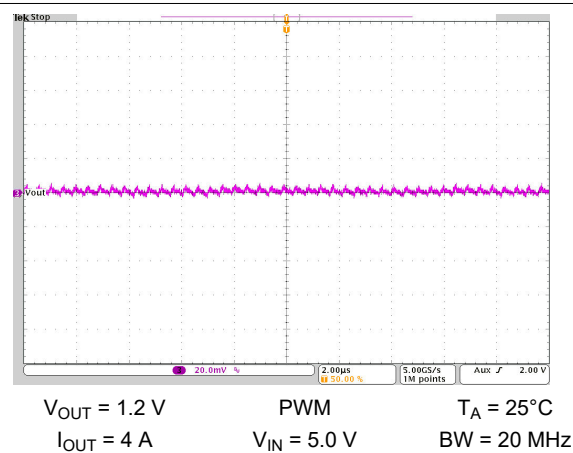
图 10-47. Output Voltage Ripple
