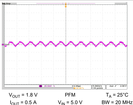
图 10-44. Output Voltage Ripple
