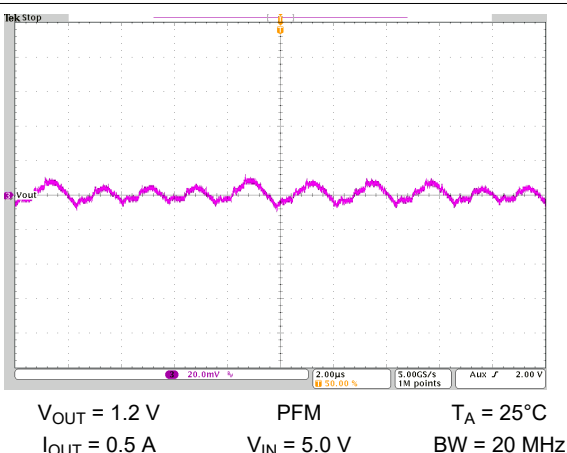
图 10-46. Output Voltage Ripple
