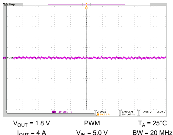
图 10-45. Output Voltage Ripple
