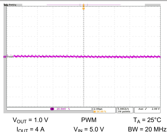
图 10-49. Output Voltage Ripple
