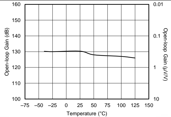
图 20. 开环增益与温度间的关系
