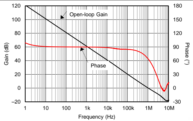
图 18. 开环增益和相位与频率间的关系
