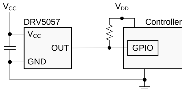
典型原理图
