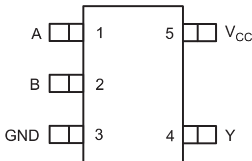
DCK 或 DBV 封装 (顶视图)
