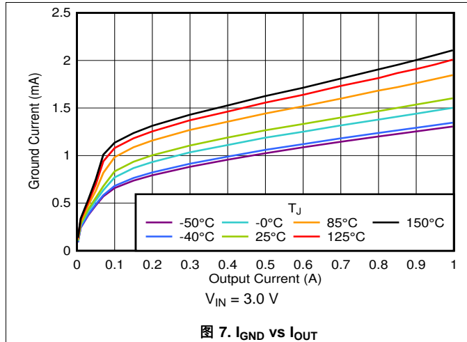
图 7. I_{GND} vs I_{OUT}
