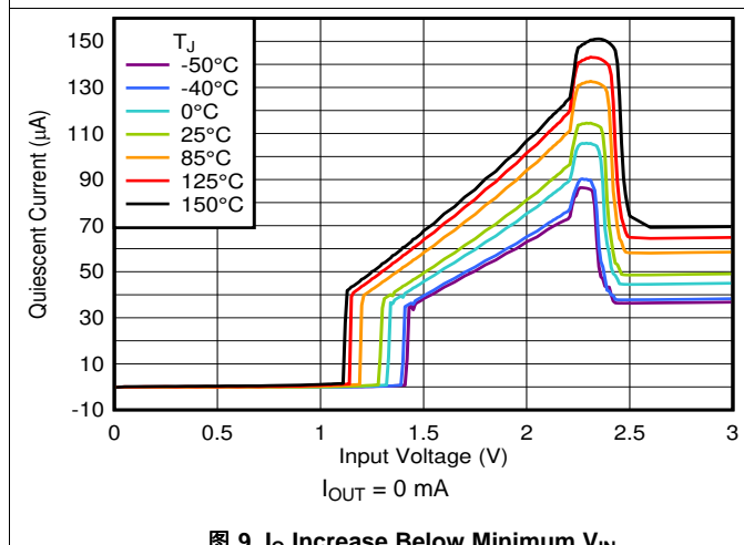
图 9. I_Q Increase Below Minimum V_{IN}
