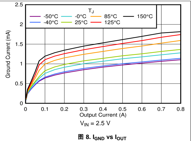
图 8. I_{GND} vs I_{OUT}
