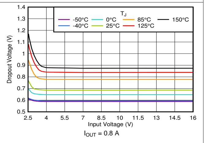
图 16. V_{DO} vs V_{IN}
