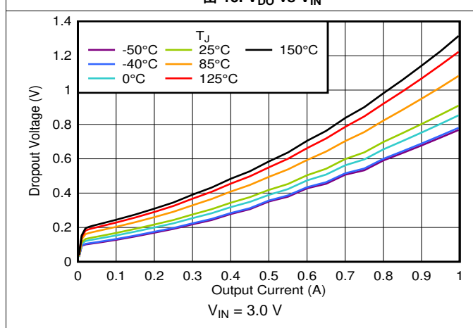
图 17. V_{DO} vs I_{OUT}
