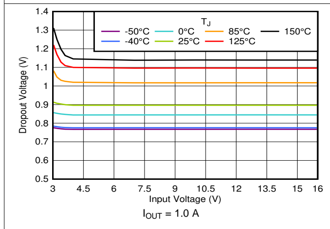
图 15. V_{DO} vs V_{IN}
