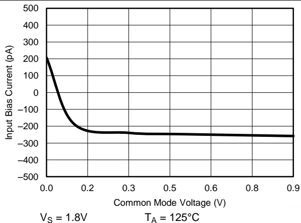
Figure 11. 输入偏置电流与共模电压间的关系
