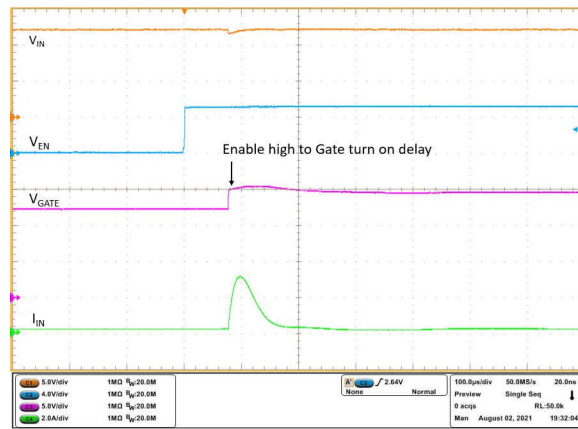
图 9-11. Enable Turn ON Delay
