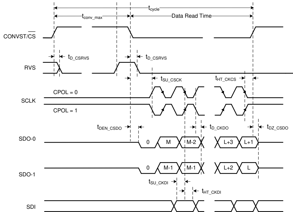
图 6-6. multiSPI 接口时序图 for Dual SDO-x 和 CPHA = 1
