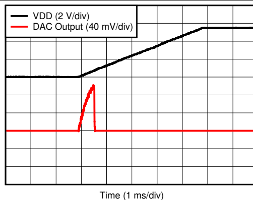
图 40. Power-on Glitch
