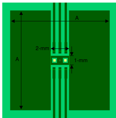
图 8-7. Board parameters used for simulation
