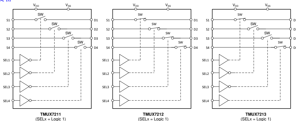
TMUX721x 方框图
