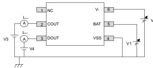
图 8-6. Test Circuit 4
