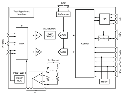
简化框图
