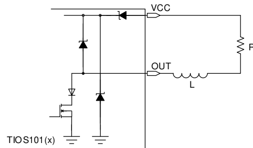
图 9-3. NPN Mode
