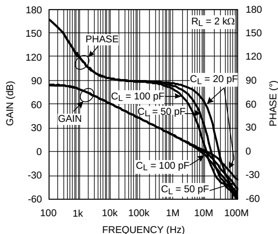
图 18. 带容性负载的开环增益和相位
