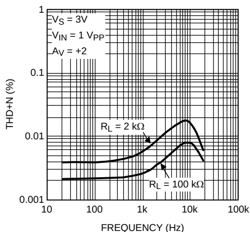
图 26. THD+N 与频率间的关系
