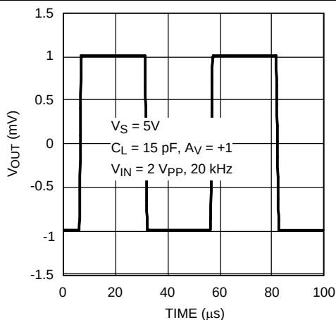
图 30. 大信号瞬态响应
