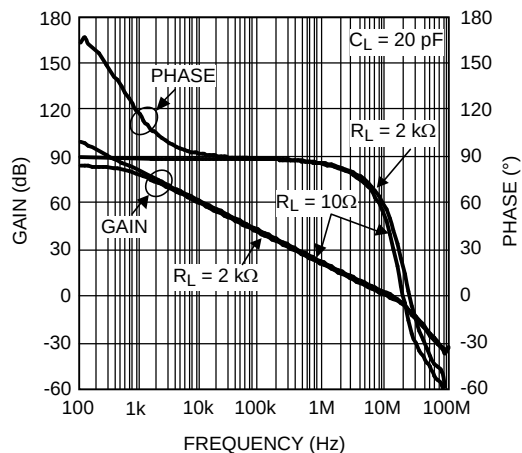
图 19. 开环增益和相位随阻性负载的变化
