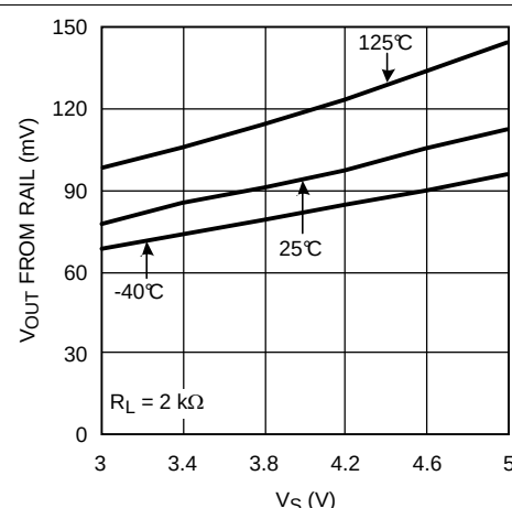
图 10. 正输出摆幅与电源电压间的关系
