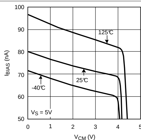
图 8. I_{BIAS} 与 V_{CM} 间的关系
