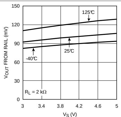
图 11. 负输出摆幅与电源电压间的关系
