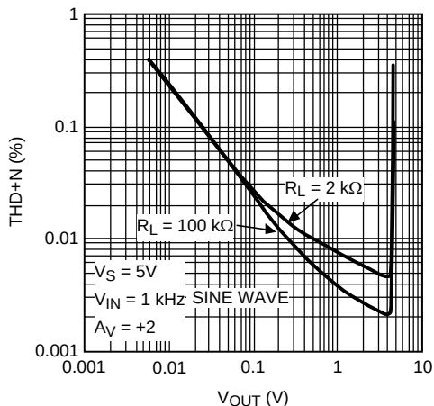
图 25. THD+N 与 V_{OUT} 间的关系
