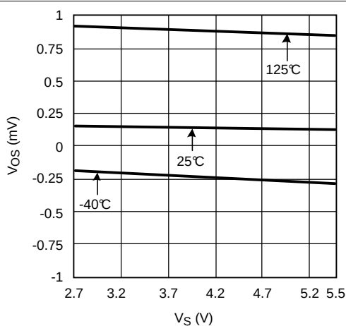
图 6. V_{OS} 与电源电压间的关系
