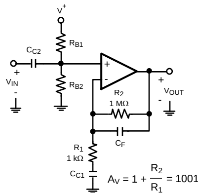
图 39. 高增益同相放大器
