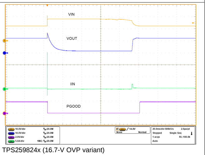
图 30. Overvoltage Protection
