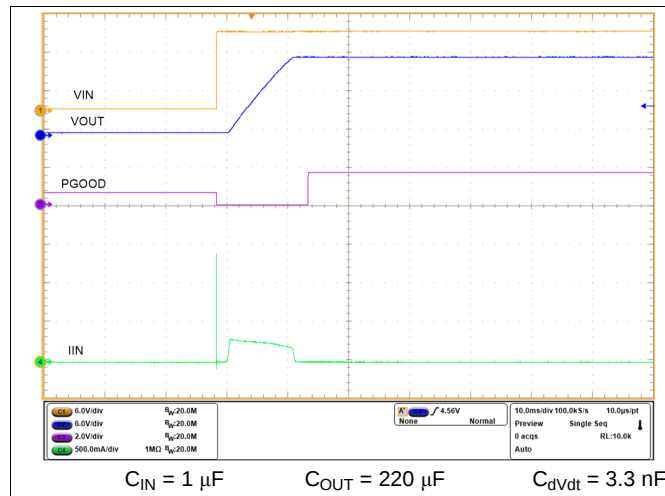
图 27. Hotplug
