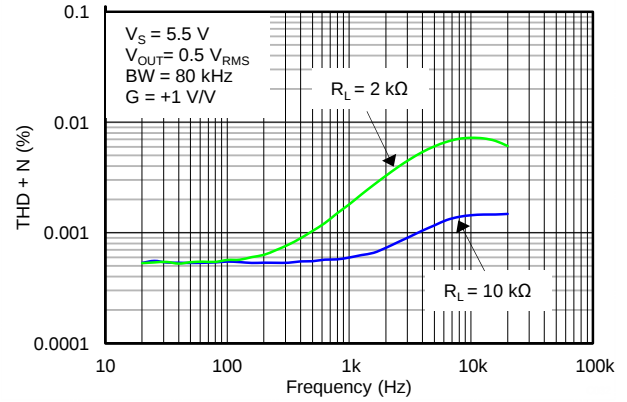
Figure 32. THD+N 与频率间的关系
