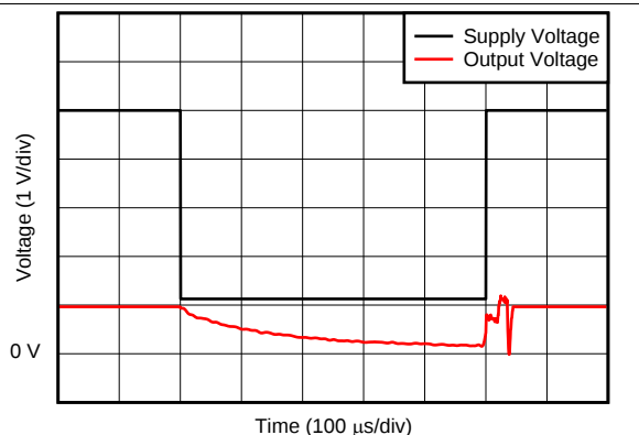
图 25. Brownout Recovery
