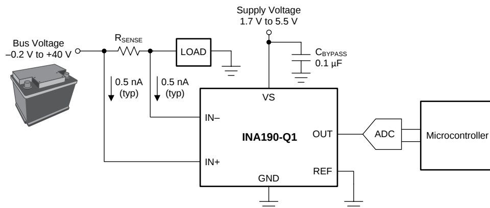
典型应用
