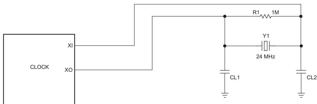
图 2. TUSB8044A Clock
