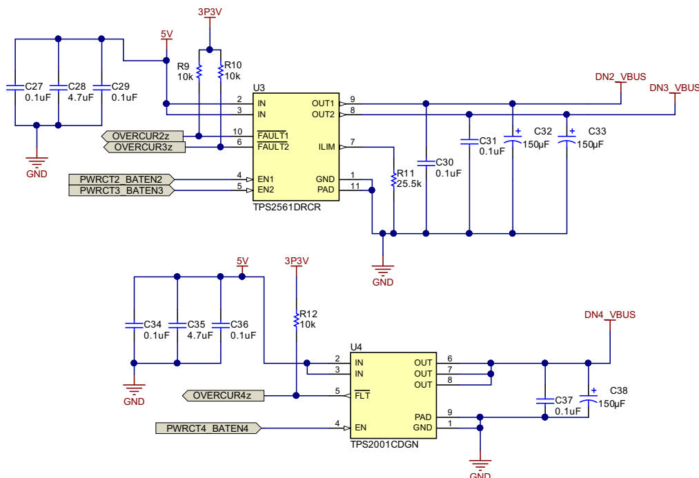
图 42. VBUS Power Switch Implementation
