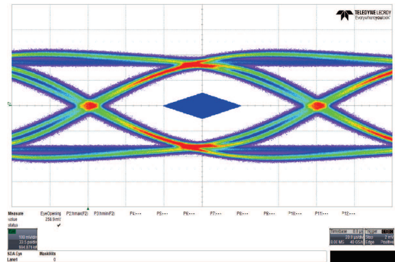
图 49. Downstream Port 1
