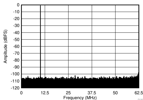
f_S = 125\text{MSPS} 、 f_{IN} = 10\text{MHz} 时的性能 ( \text{SNR} = 70.6\text{dBFS} , \text{SFDR} = 100\text{dBc} )
