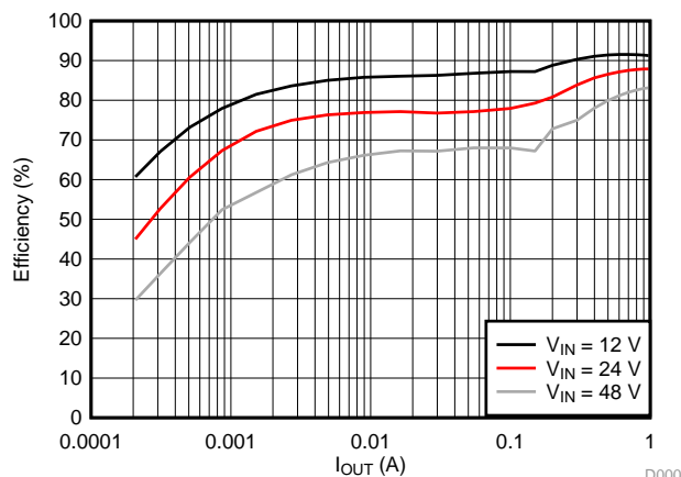
效率与输出电流间的关系 ( V_{out} = 5\text{V} , f_{sw} = 500\text{kHz} )
