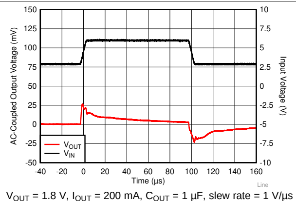
图 24. V_{IN} Transient From 2.8 V to 6.0 V
