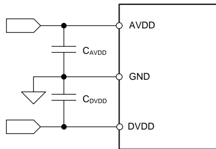
图 49. Power-Supply Decoupling
