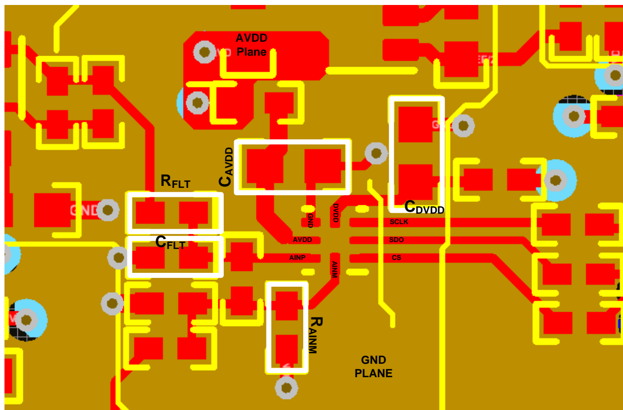
图 51. Example Layout
