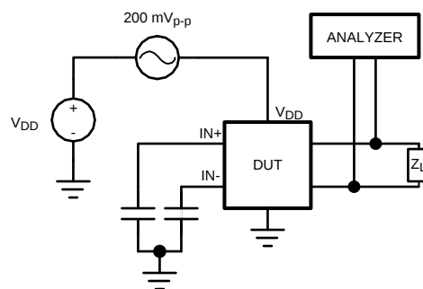
图 12. PSRR Test Circuit
