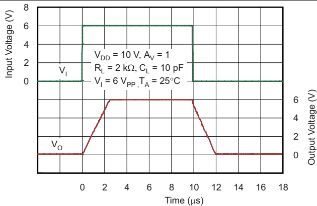
图 19. 电压跟随器大信号 脉冲响应
