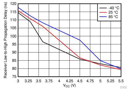
D002_rx_tpLH.grf
