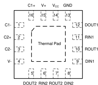
图 5-2. RGT, VQFN Package (Top View)
