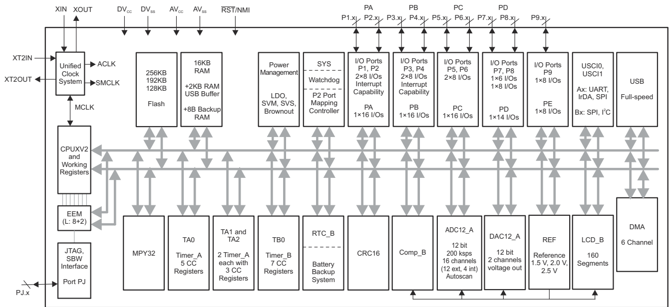
图 4-1. 功能框图 - MSP430F6638、MSP430F6637 和 MSP430F6636
