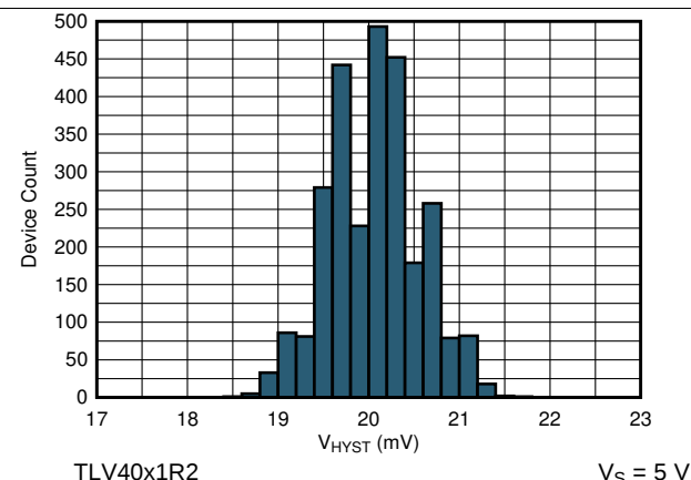
图 14. Hysteresis Histogram
