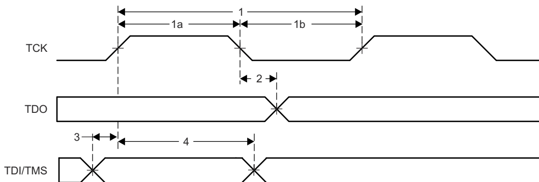
图 7-19. JTAG Timing
