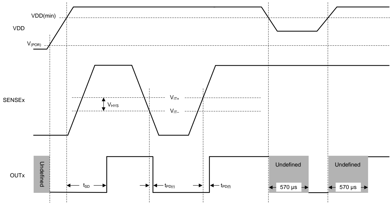
图 1. Timing Diagram
