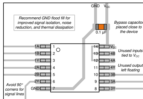
图 11. Example layout for the SN74HCS86-Q1
