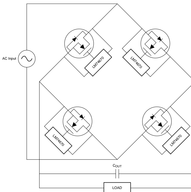
智能二极管全桥整流器应用
