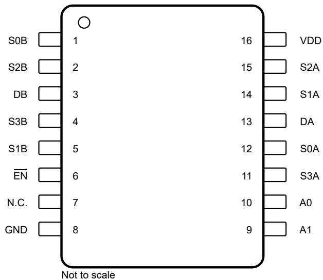
图 6-4. TMUX1309-Q1: PW Package 16-Pin TSSOP Top View
