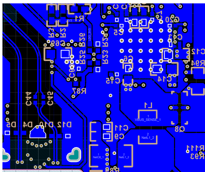
图 12-10. Top Layer Component Routing
