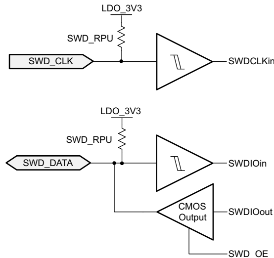
图 9-51. IOBUF_GPIOHSSWD
