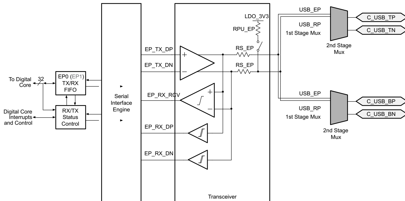
图 9-38. USB Endpoint Phy
