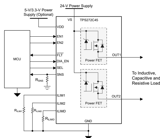
典型应用原理图
