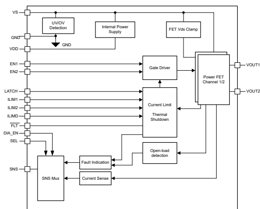
功能方框图
