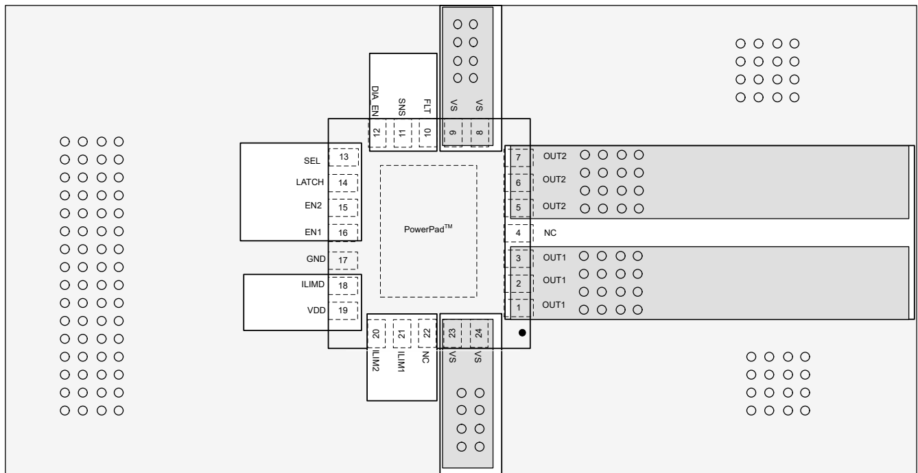
图 12-1. Layout Example
