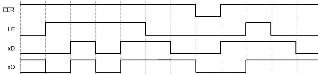
图 6-1. Timing Diagram
