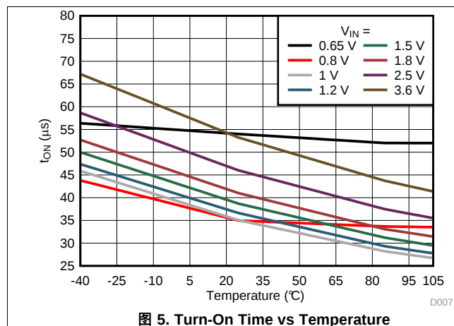
图 5. Turn-On Time vs Temperature
