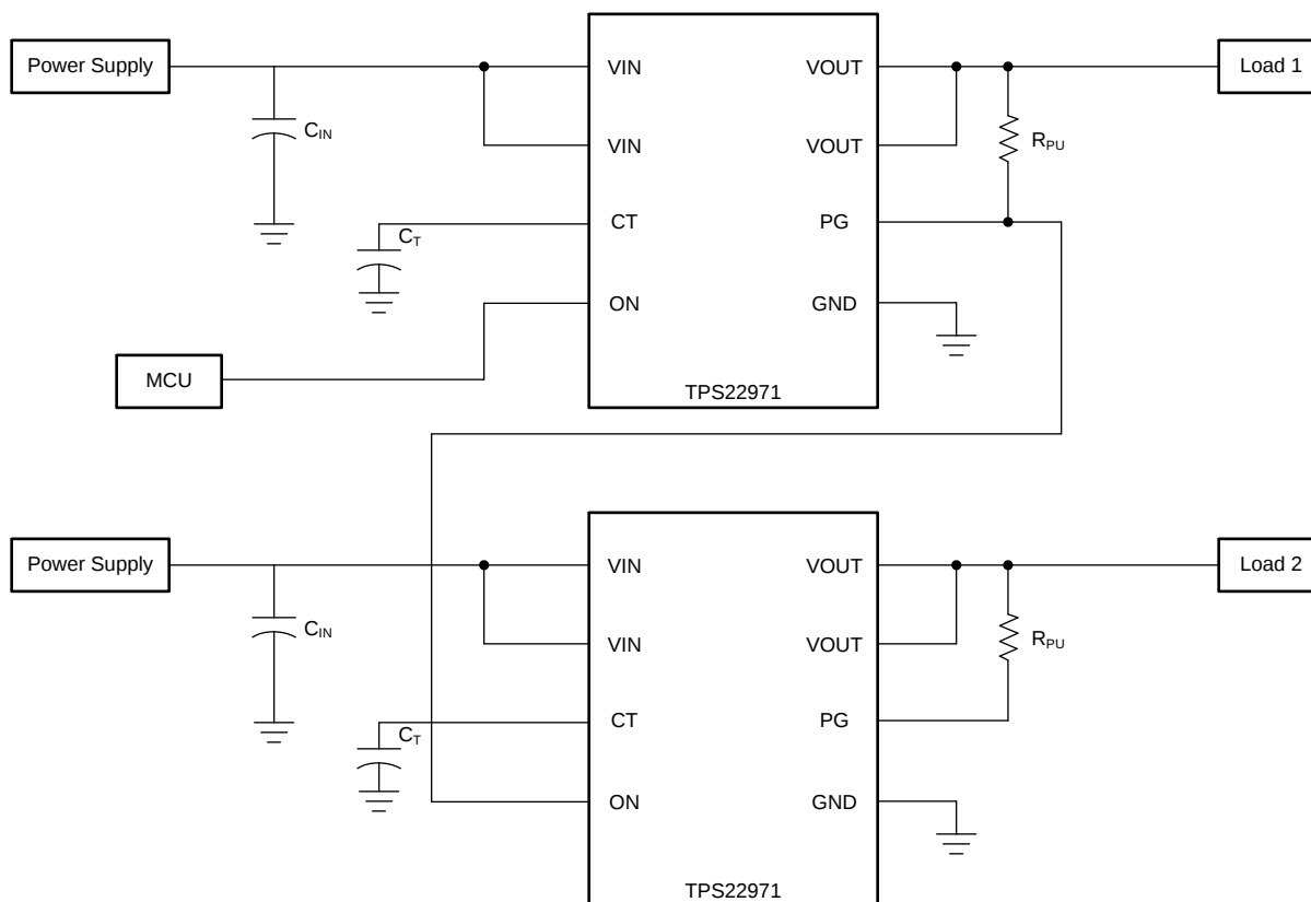
图 26. Power Sequencing
