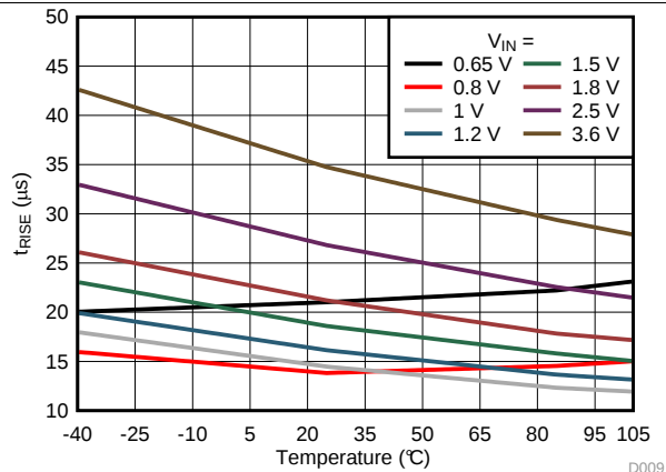
图 7. Rise Time vs Temperature
