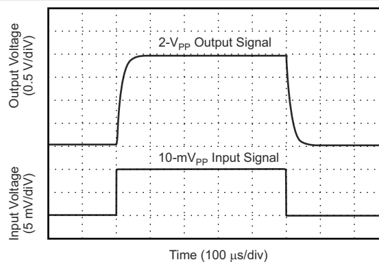
图 7-14. Step Response (10-mV pp Input Step)
