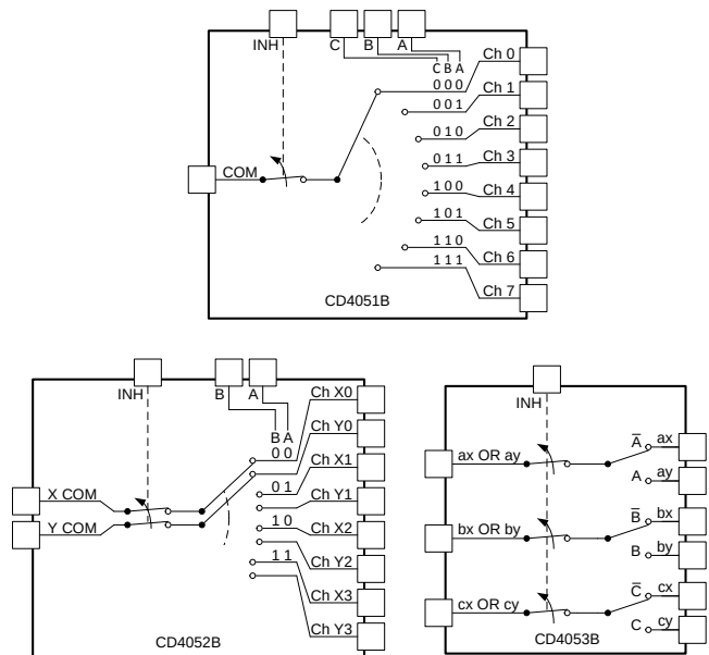
CD405xB-Q1 的功能图
