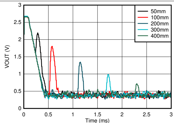
图 30. TUS4470 400 kHz Ranging at 5-V Drive
