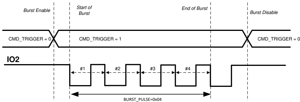
图 15. IO_MODE 0 Description
