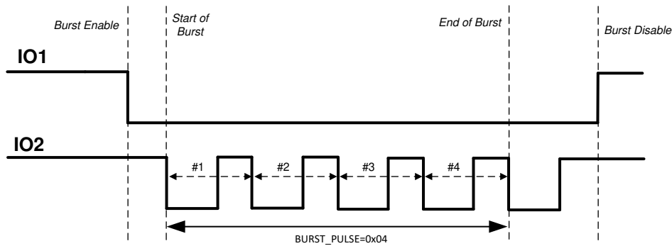
图 16. IO_MODE 1 Description
