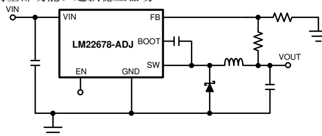
简化版应用电路原理图
